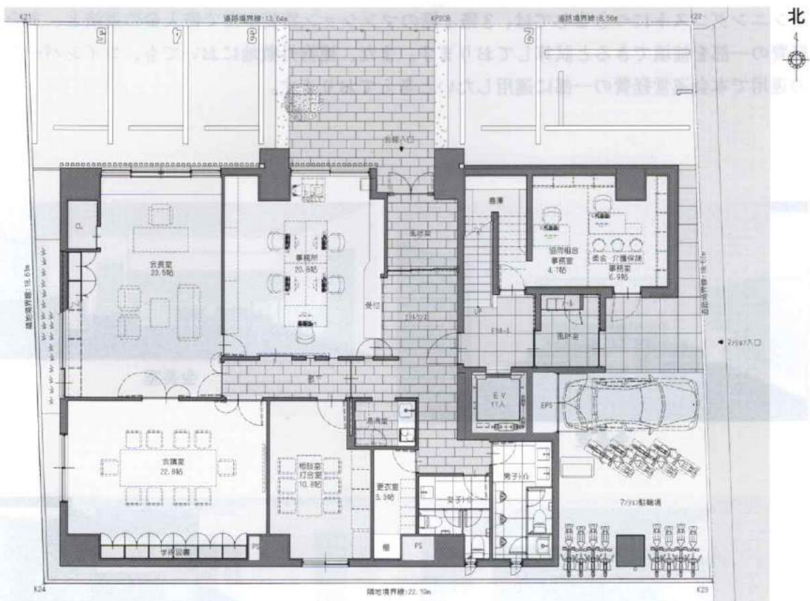
1階平面図
