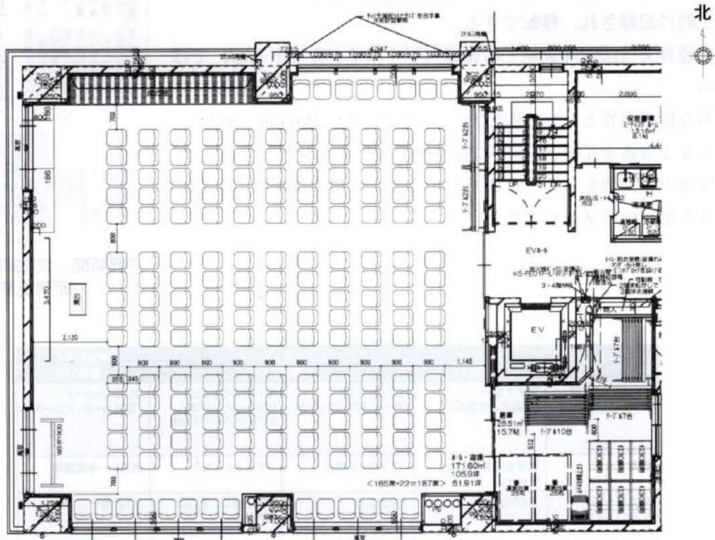
2階レイアウト 椅子のみ
